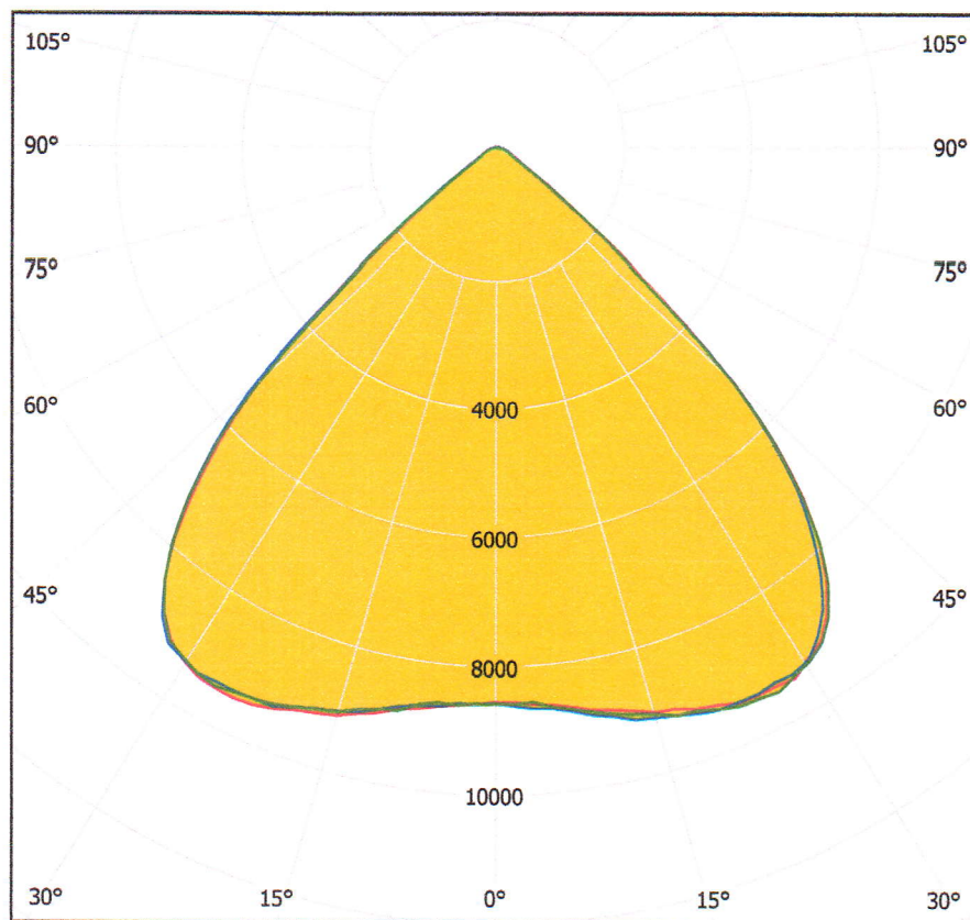
Рисунок 1 – КСС образца светильник светодиодный ДСП-04-120-5KK-20400-Г90-IP66 в поперечной (С0-С180) (красная кривая), продольной (С90-С270) (синяя кривая) плоскостях и плоскости максимальной силы света (С182-С2) (зеленая кривая)
