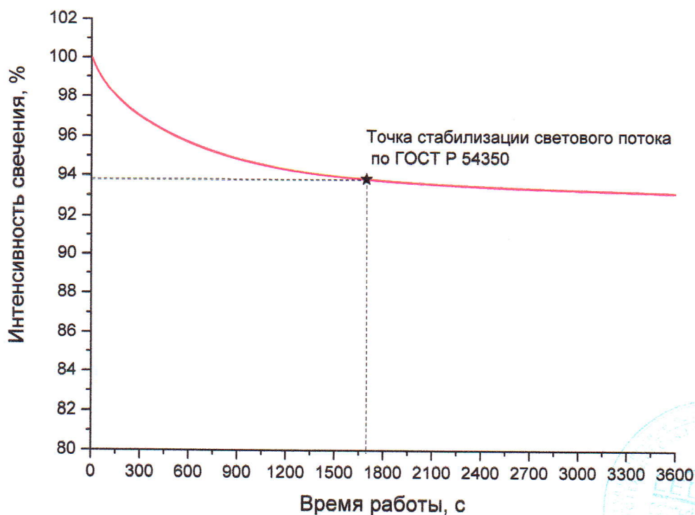
Рисунок 2 – График стабилизации светового потока образца светильник светодиодный ДСП-04-120-5KK-20400-Г90-IP66
