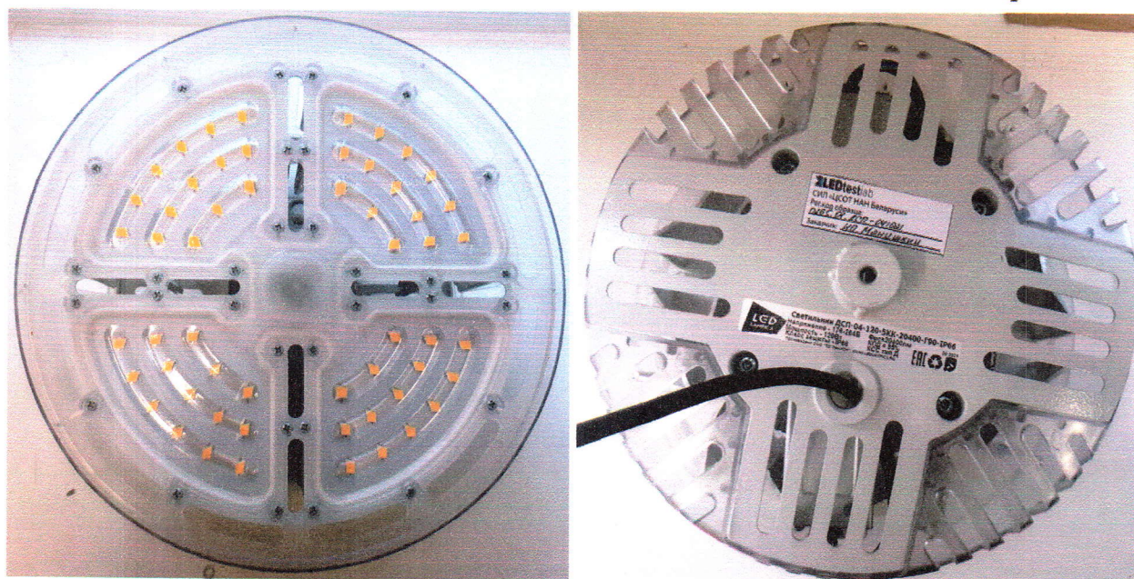
Рисунок 4 – Фотографии образца светильник светодиодный ДСП-04-120-5КК-20400-Г90-IP66
